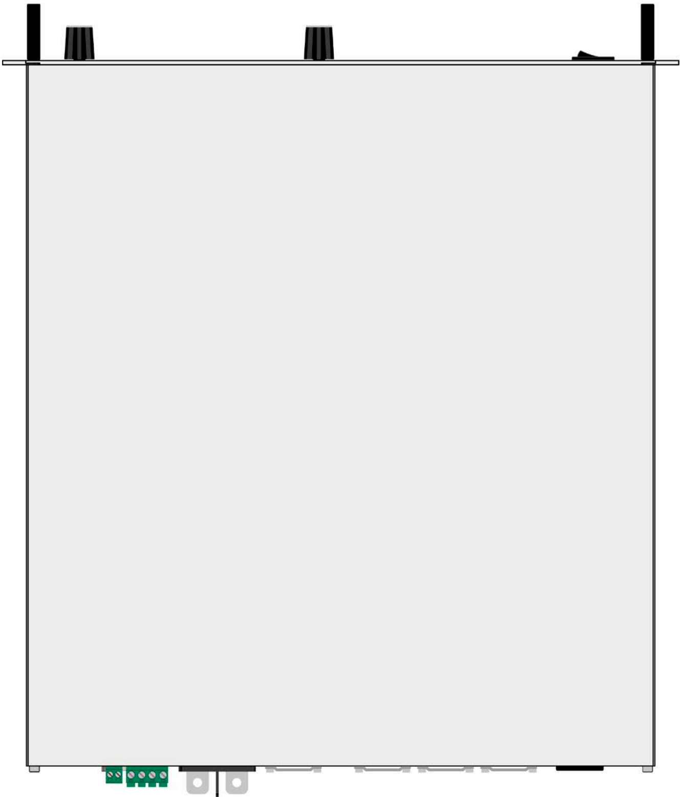
图 5 - 俯视图
