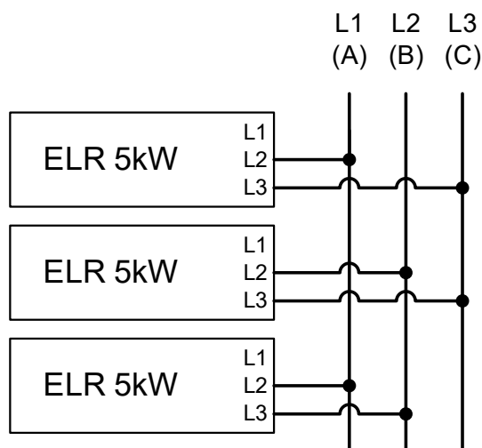
Figure 8 - Exemple de câblage AC équilibré d'unités 5 kW
