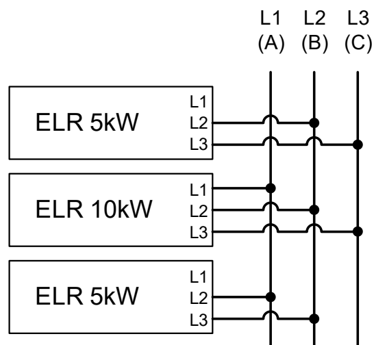
Figure 9 - Exemple de câblage AC pour plusieurs unités avec des puissances différentes et courant quasi-équilibré
