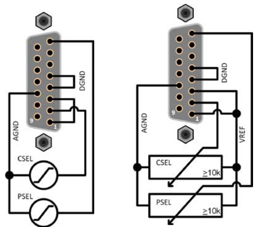
Beispiel mit ext. Spannungsquelle
