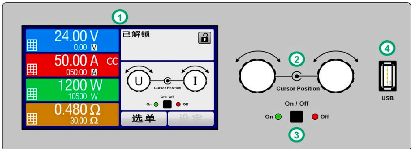
图 6 - 控制面板
