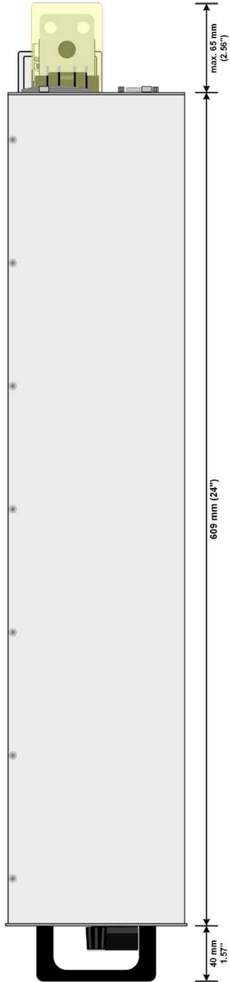
图 4 - 右侧视图
