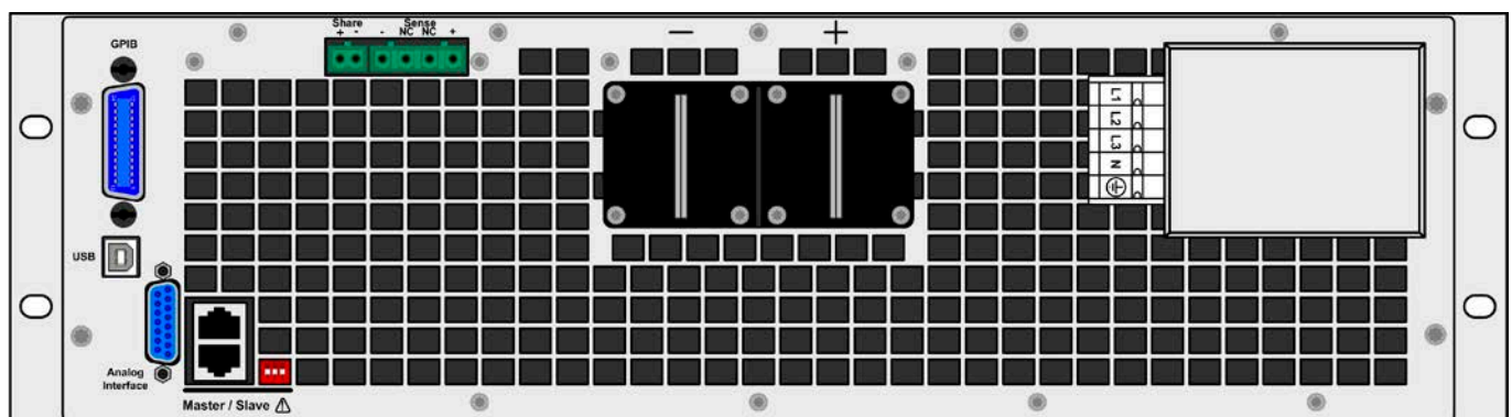
Rückansicht mit Option 3W ( GPIB)
