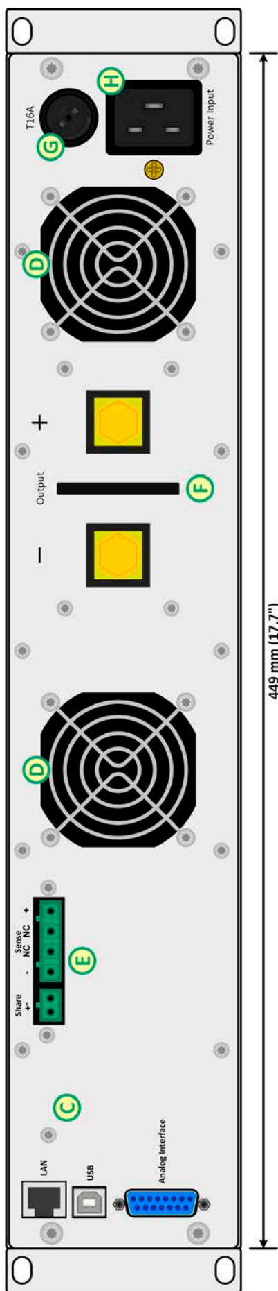
Bild 2 - Rückseite (Standardausführung)
