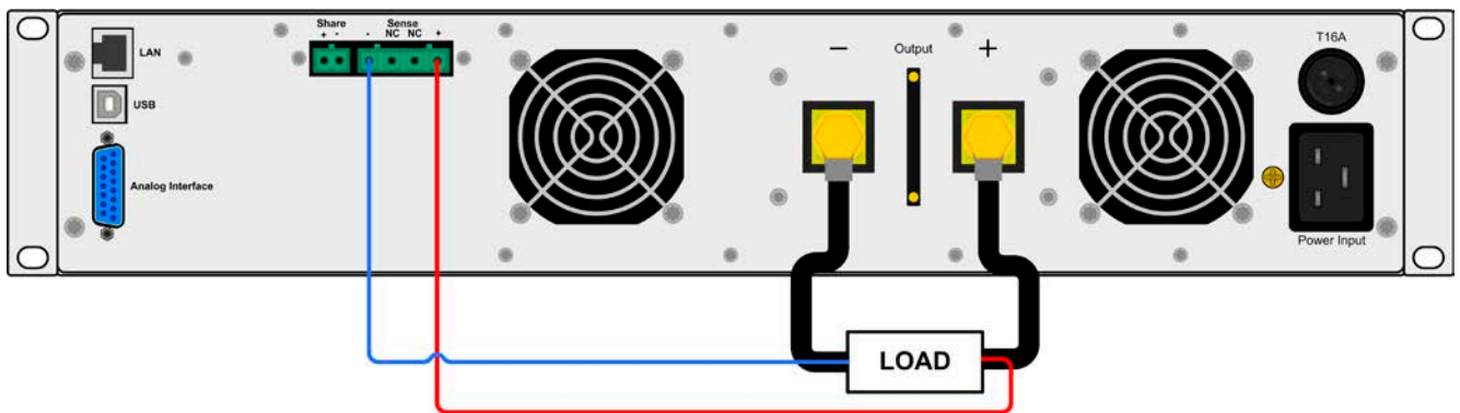
Bild 7 - Beispiel Fernfühlungsverdrahtung
