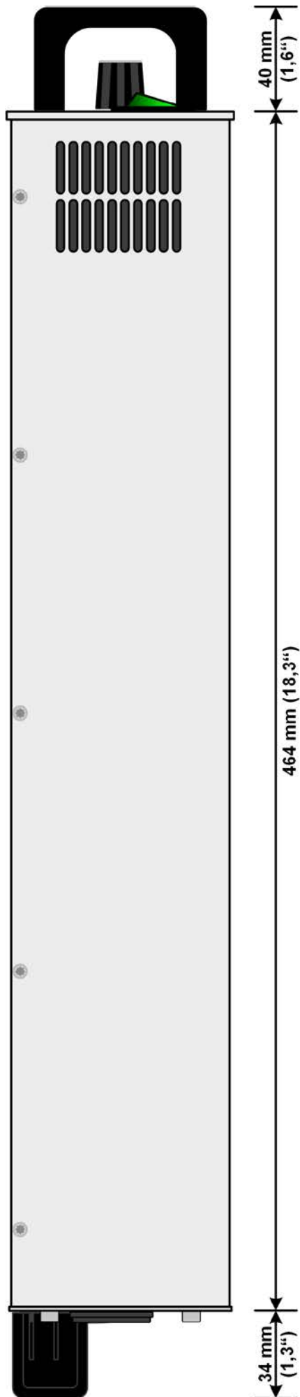
Figure 3 - Vue de côté (gauche) avec couvercle DC
