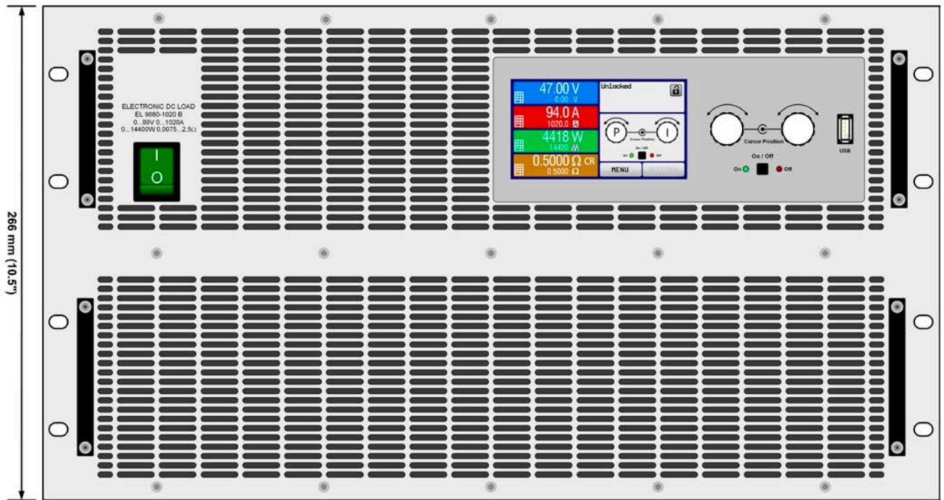
图 6 - 前视图
