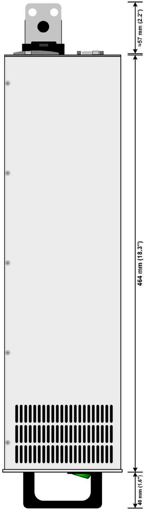
图 4 - 右侧视图, 不带直流端子盖
