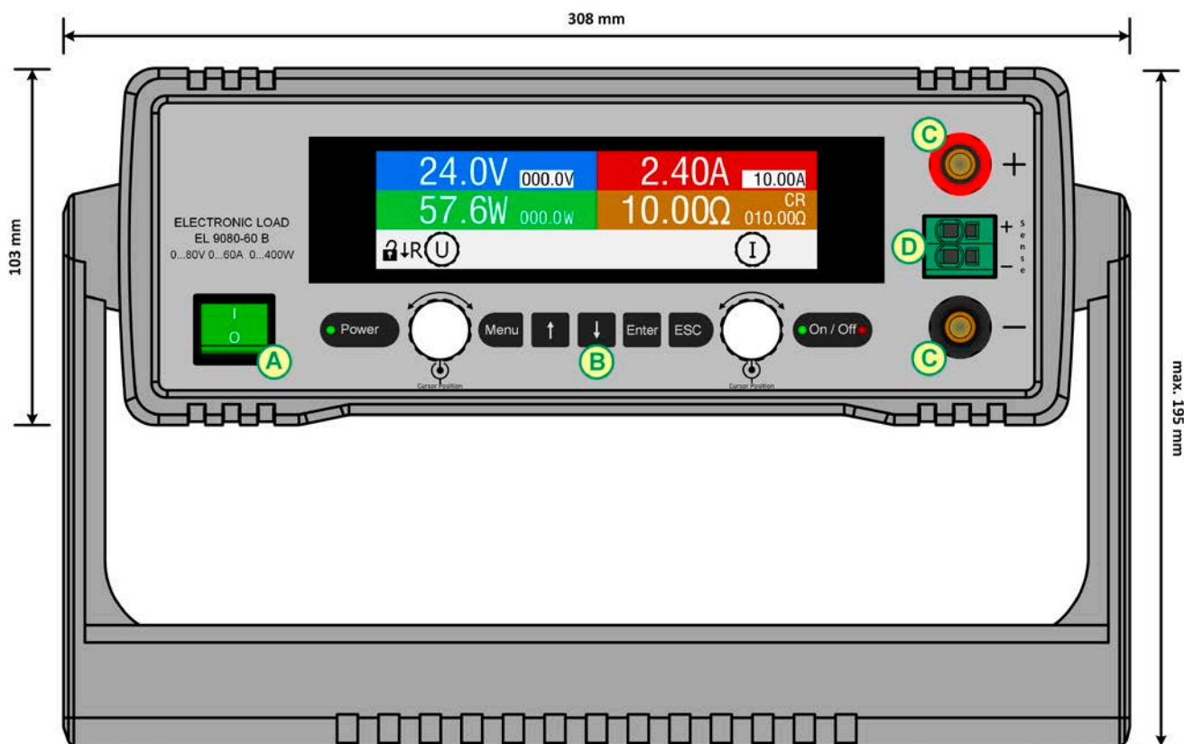
图 1 - 前视图
