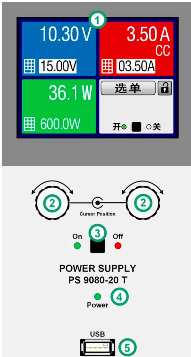
图 6 - 控制面板
