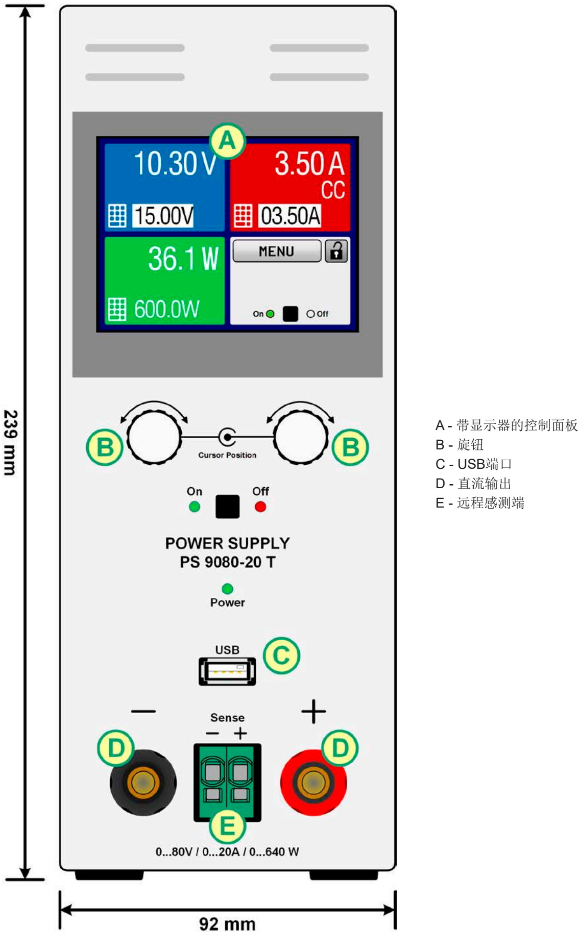
图 1 - 前视图
