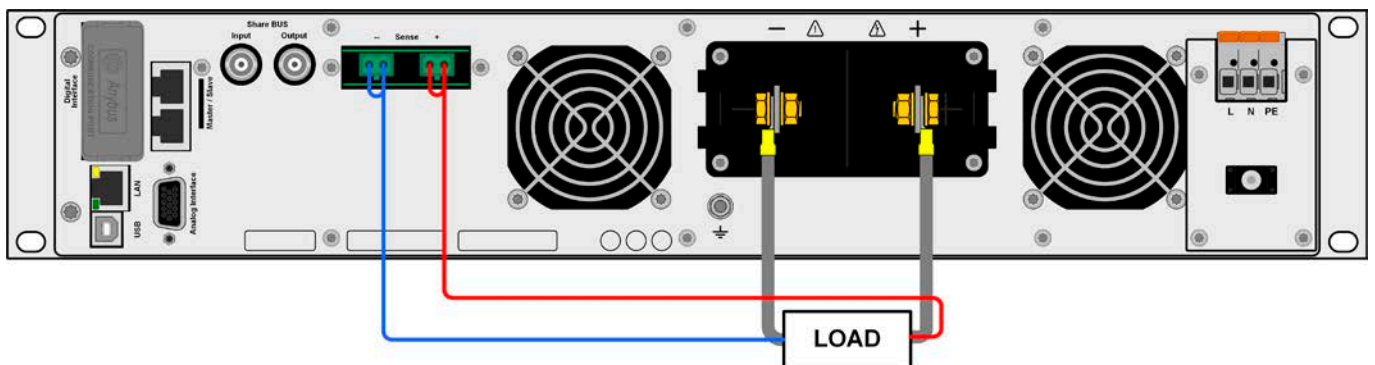
Figure 13 - Exemple de câblage de mesure à distance (bornier DC et Sense couvrent la voie de gauche à des fin d'illustration) Schémas de branchement autorisés
