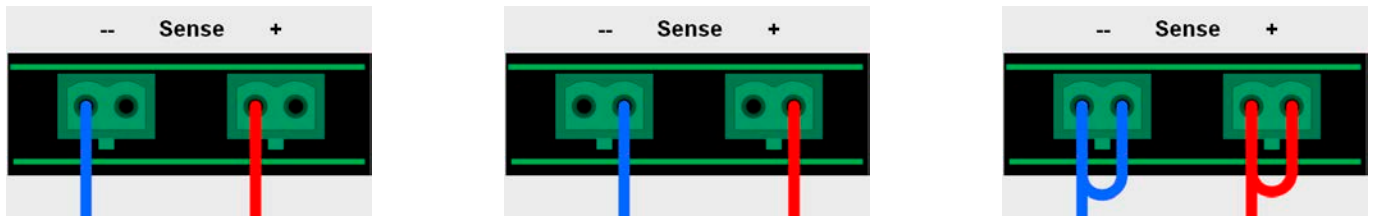
Figure 13 - Exemple de câblage de mesure à distance (bornier DC et Sense couvrent la voie de gauche à des fin d'illustration) Schémas de branchement autorisés
