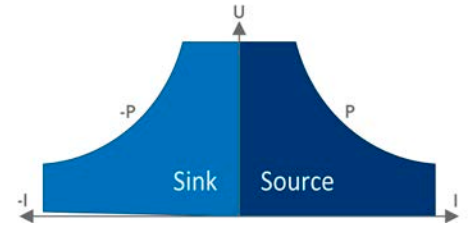
Figure 14 - Gamme de puissance des modèles 60 V
