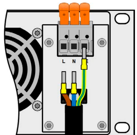
Figure 10 - Exemple de configuration câble AC
