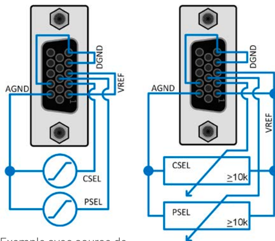
Exemple avec source de tension externe
