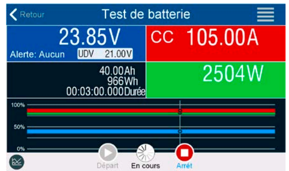
Figure 16 - Exemple de décharge statique
