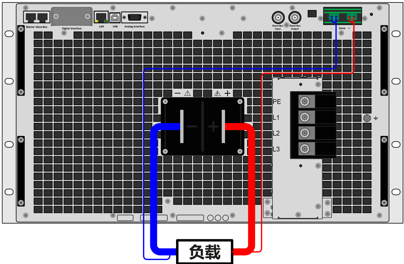
图 13 - 远程感测接线示例 (为了清晰展示接线, 不使用直流端子和感应端子罩)
