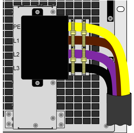
图 11 - 完整的交流端
