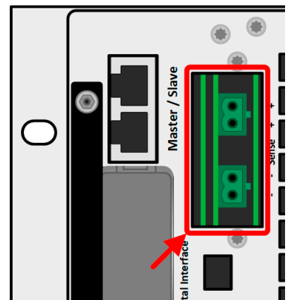
图 6 - 远程感测连接器
