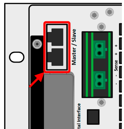
图 7 - 主从总线端口
