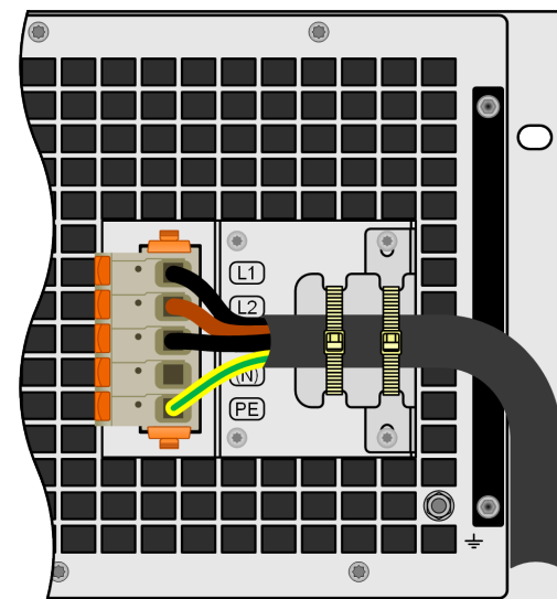
图 12 - 完整安装的固定支架
