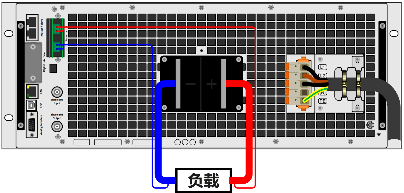
图 14 - 远程感测接线示例 (为了清晰展示接线, 没有加上直流端子和感应端子罩)
