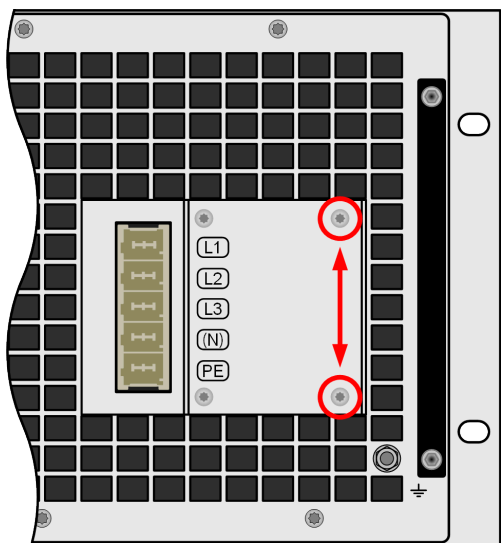
图 11 - 支架的安装位置
