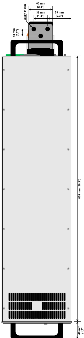
所示为风冷型设备的侧视图
