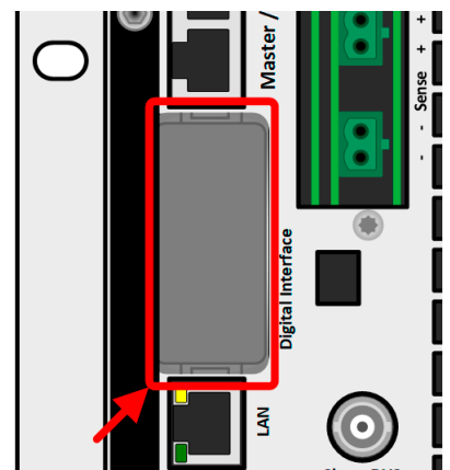
图 3 - 接口插槽
