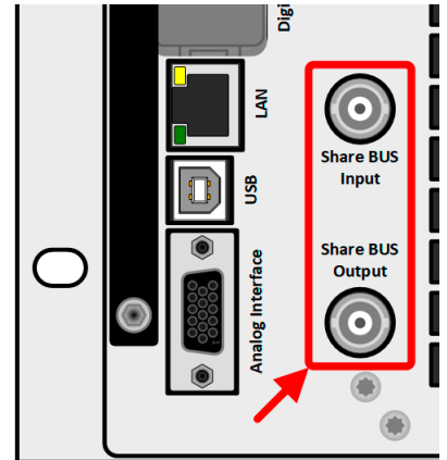
图 5 - 共享总线
