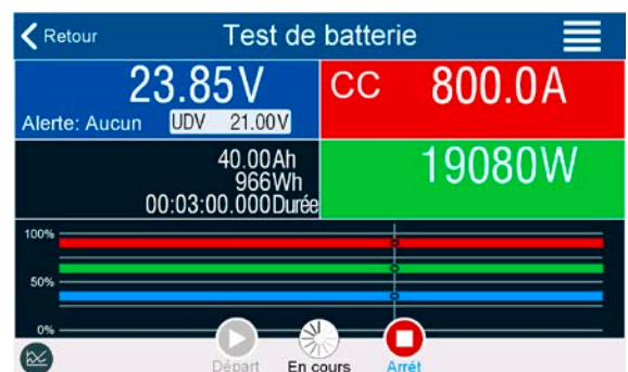
Figure 16 - Exemple de décharge statique
