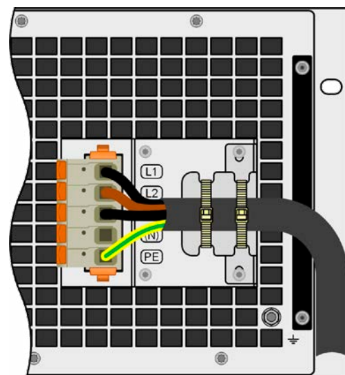
Figure 12 - Bride de soulagement entièrement montée
