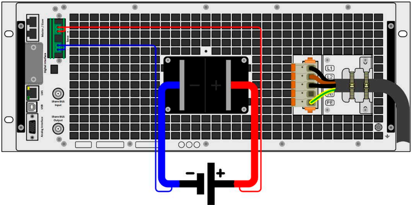
Figure 14 - Exemple de câblage de mesure à distance (borniers DC et Sense couvrent la voie de gauche à des fin d'illustration)
