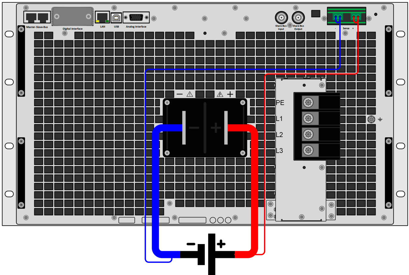
图 14 - 远程感测接线示例（为了清晰展示接线，不使用直流端子和感应端子罩）
