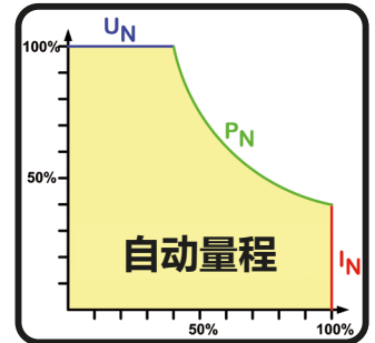
图 15 - 功率范围
