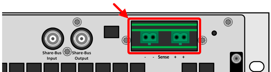
图 6 - 远程感测端子
