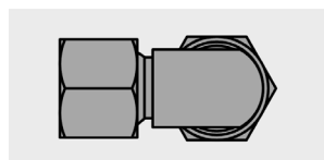
龙头: 10 mm 软管, M19 螺母
