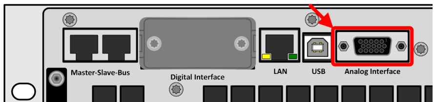
图 4 - 模拟量接口
