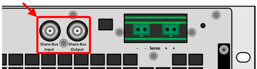
图 5 - 共享总线
