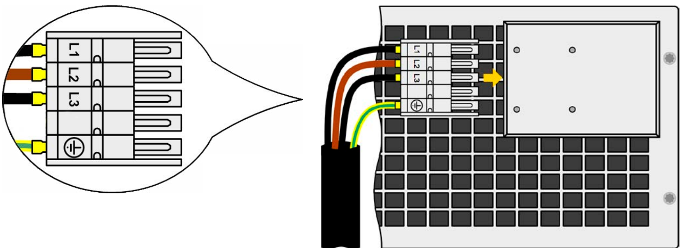
Рисунок 9 - Пример кабеля для электросети (кабель не включается в поставку)
