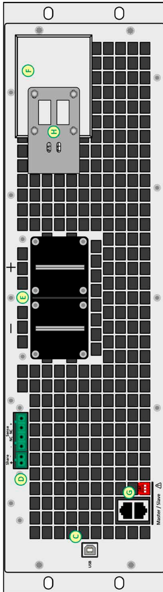
Рисунок 4 - Вид сзади (PSI 9000 WR 3U Slave)
