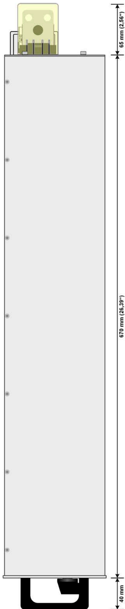
图 4 - 侧视图 (左边)
