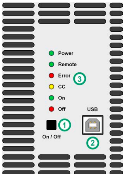
图 6 - 控制面板
