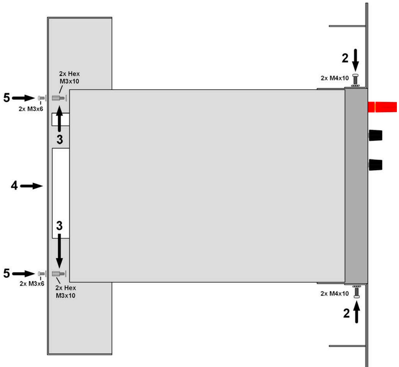
Рисунок 9 - Действия по монтажу каркаса
