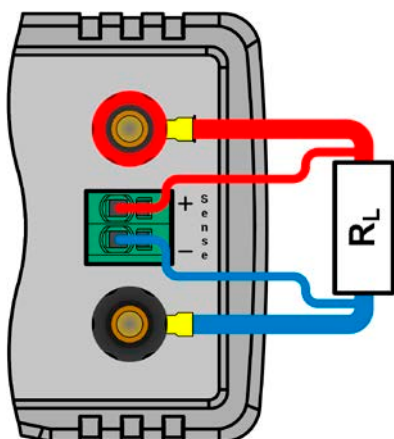
Рисунок 13 - Пример принципа соединения удалённой компенсации
