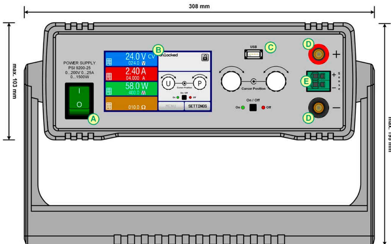
Рисунок 1 - Вид спереди (ручка для переноса в вертикальной позиции)
