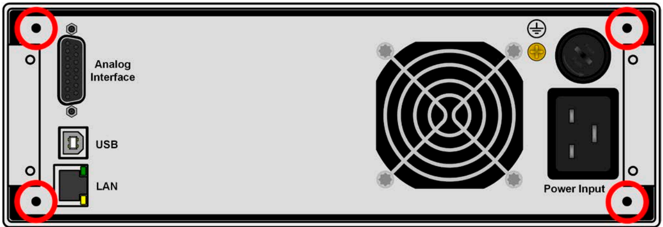
Рисунок 10 - Позиции для шестигранных втулок (3) (показана модель 1000 Вт / 1500 Вт)
