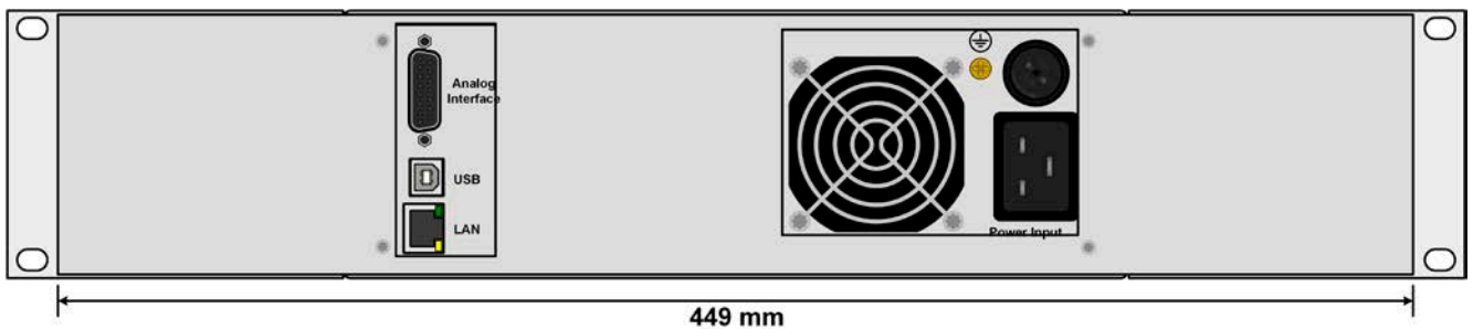
Рисунок 11 - Вид сзади после полной установки каркаса (показана модель 1000 Вт / 1500 Вт)
