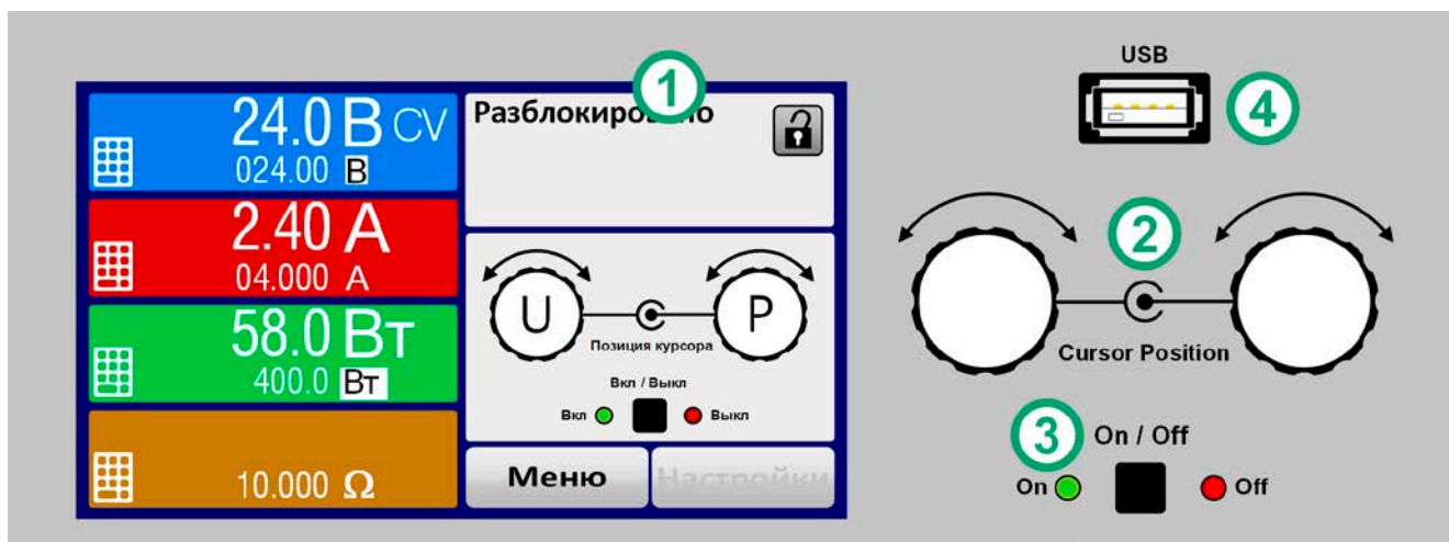
Рисунок 6 - Панель управления
