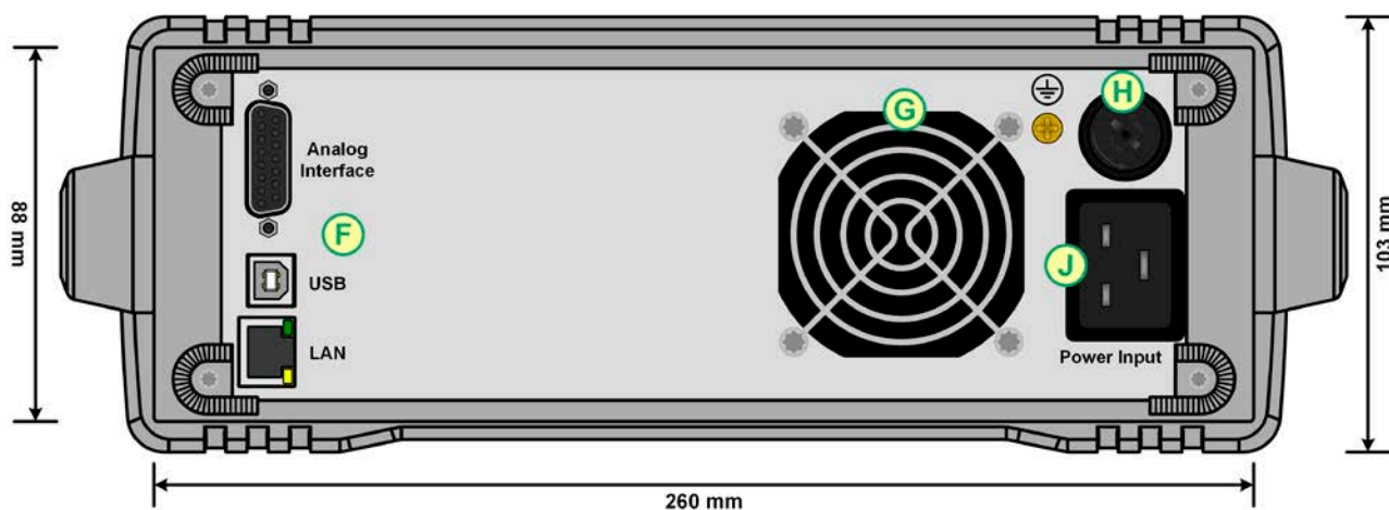
Рисунок 2 - Вид сзади (показана модель 1000 Вт / 1500 Вт)
