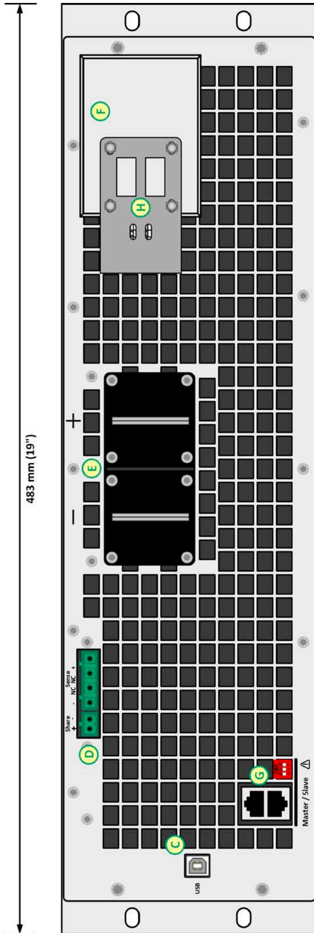
图 4 - 后视图 (PSI 9000 WR 3U Slave)
