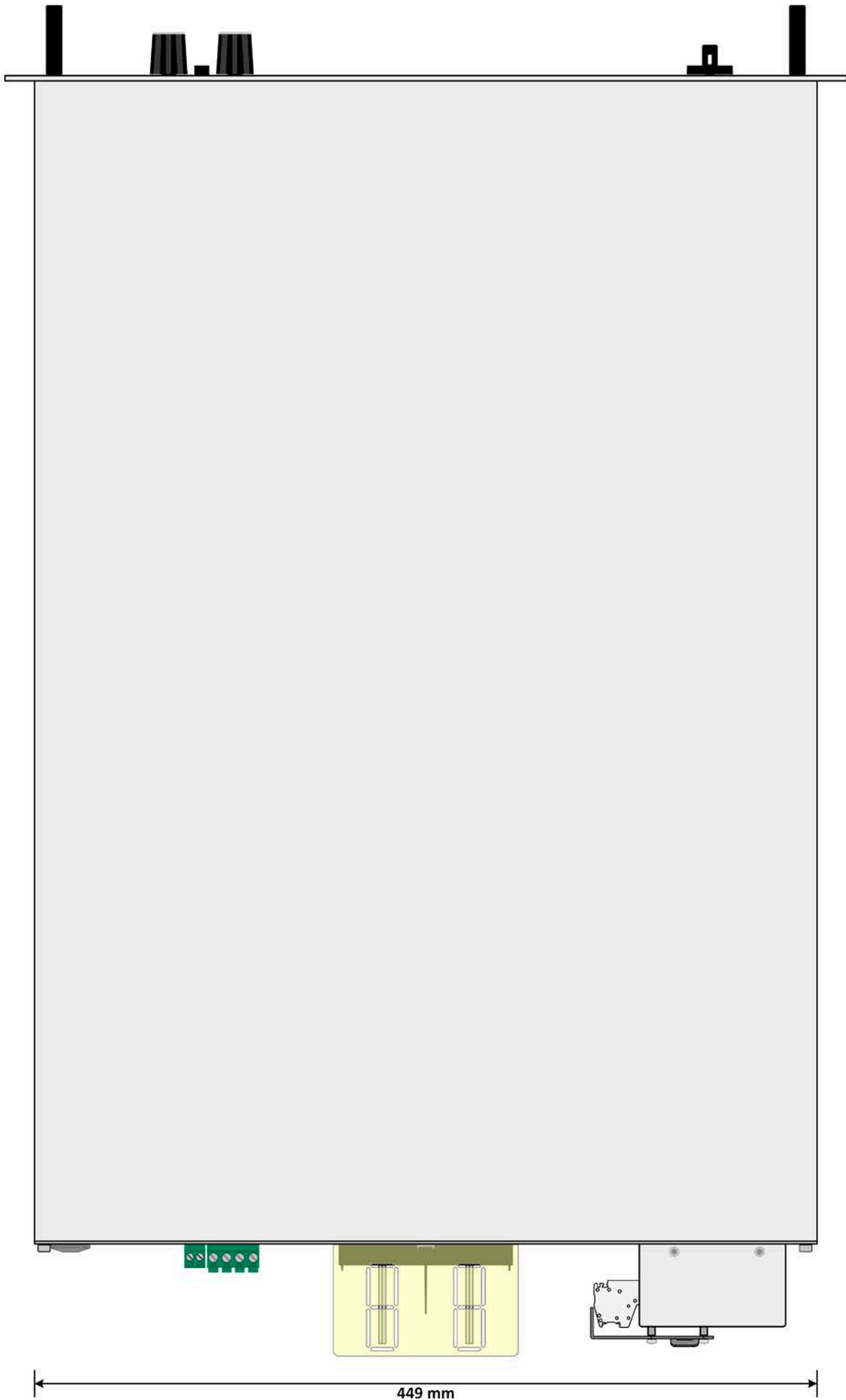
图 7 - 俯视图
