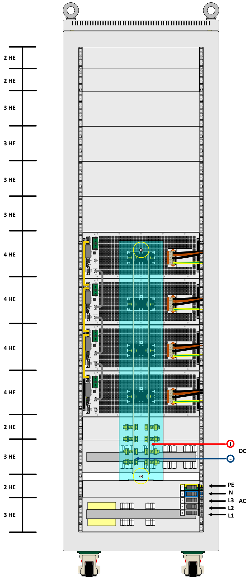
Rückansicht / Rear view
