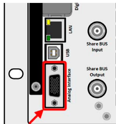
Bild 4 - Analochnittstelle
