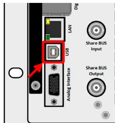
Bild 2 - USB-Port
