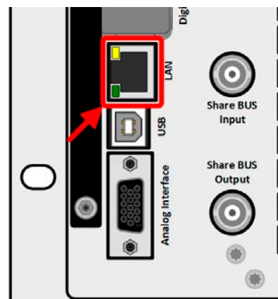
Bild 8 - LAN-Port
