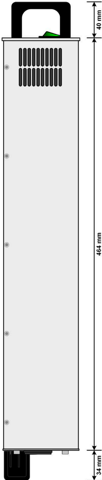
图 3 - 左侧视图, 带直流端子盖
