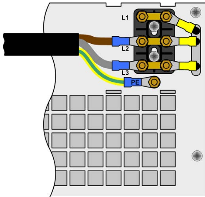
Bild 6. Netzanschluß 3.3 kW/5 kW Alle Schraubverbindungen M4
