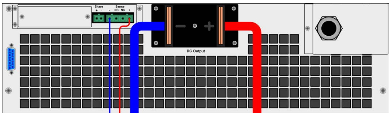
Bild 10. Verdrahtung Fernfühlung
