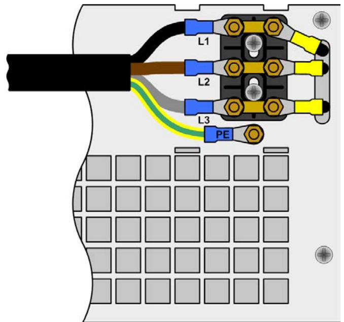
Bild 7. Netzanschluß 6.6 kW/10 kW/15 kW Alle Schraubverbindungen M4
