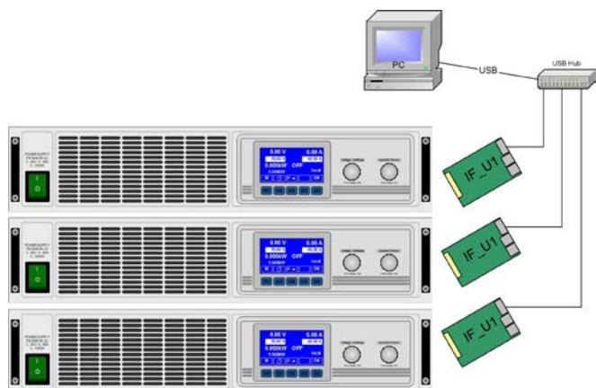
Bild 16. USB- oder RS232-Vernetzung, auch Ethernet
