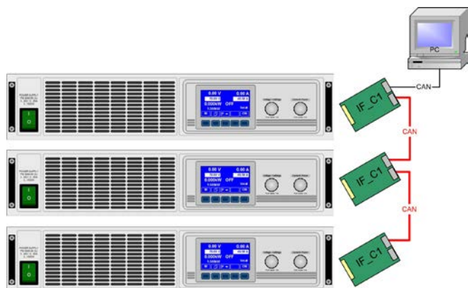
Bild 15. CAN-Vernetzungsbeispiel, gilt auch für GPIB oder Profibus
