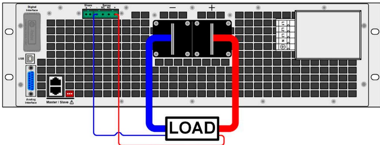
图 8 - 远程感测接线举例
