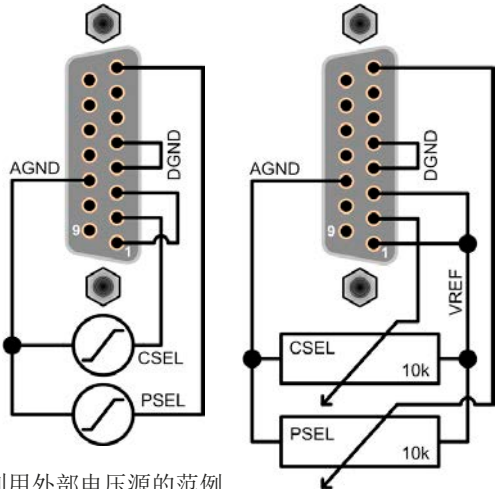
利用外部电压源的范例
