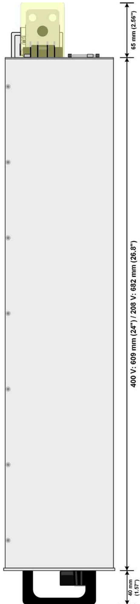
图 4 - 右侧视图
