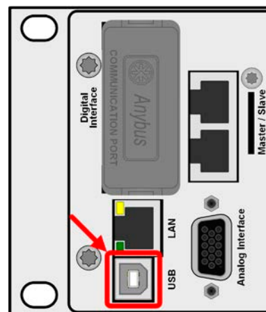
Bild 2 - USB-Anschluß
