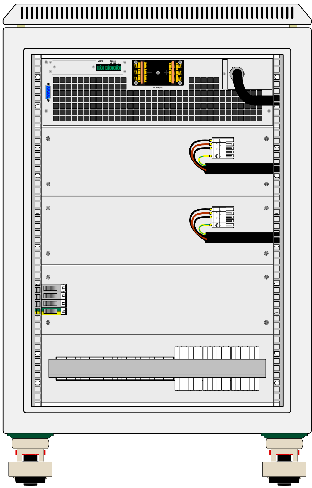
Rückansicht / Rear view
