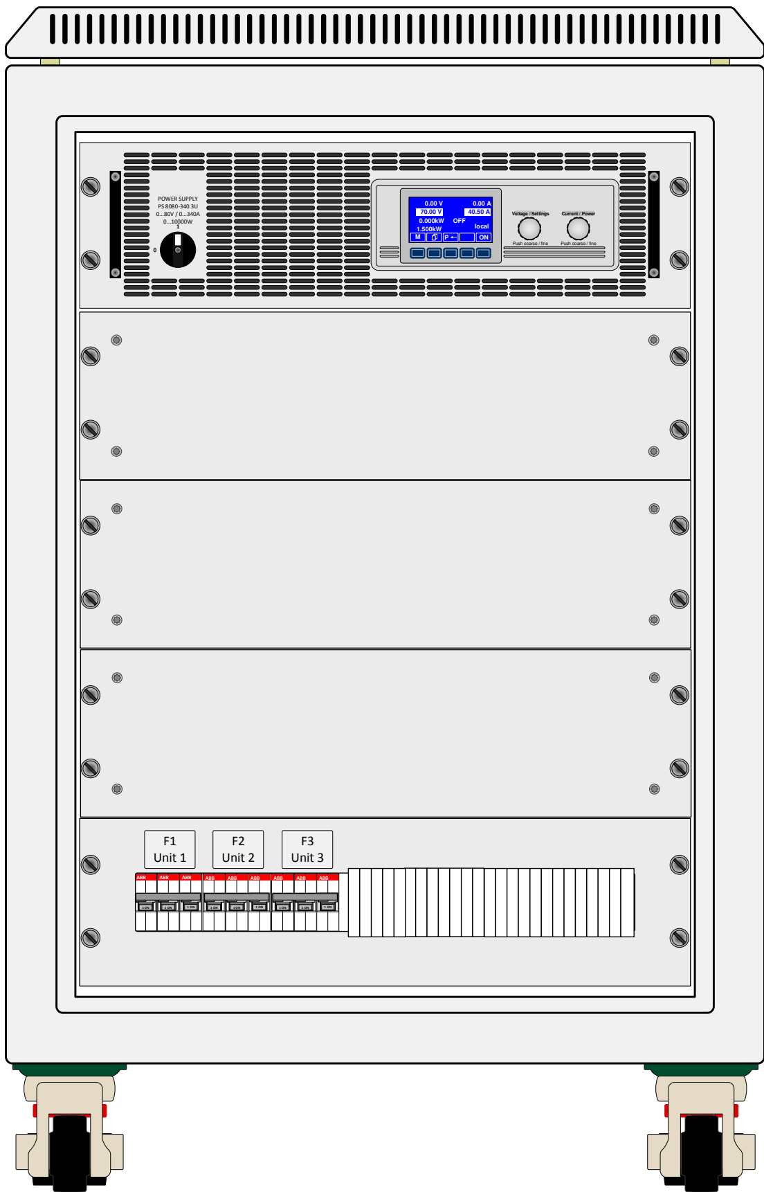
Vorderansicht mit Netzgerät / Front view with device installed
