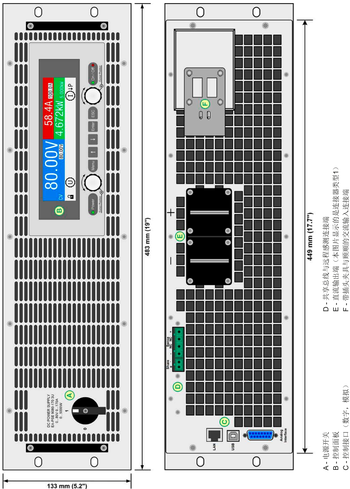
图 1 - 前视图
