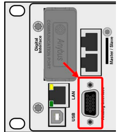
Bild 4 - Anologschnittstelle
