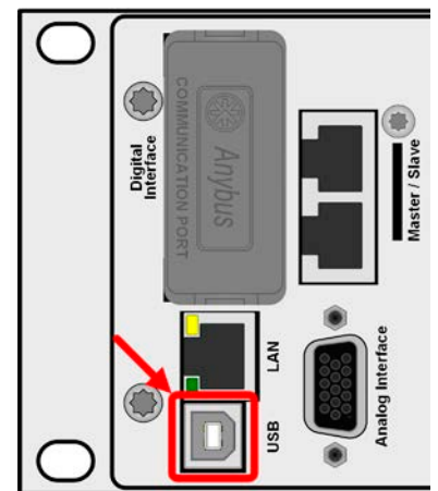
Bild 2 - USB-Port
