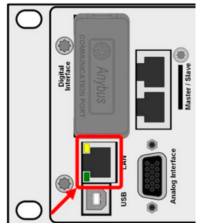
Bild 8 - LAN-Port
