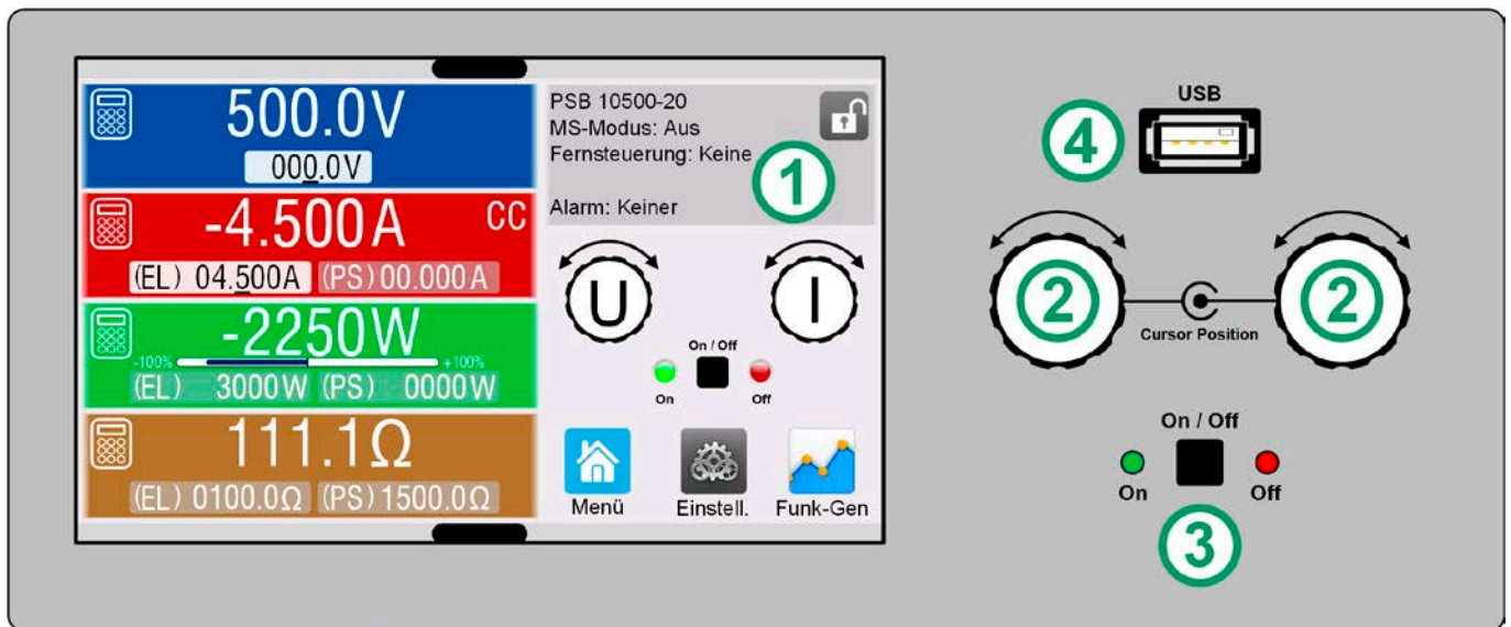
Bild 1 - Bedienfeld
