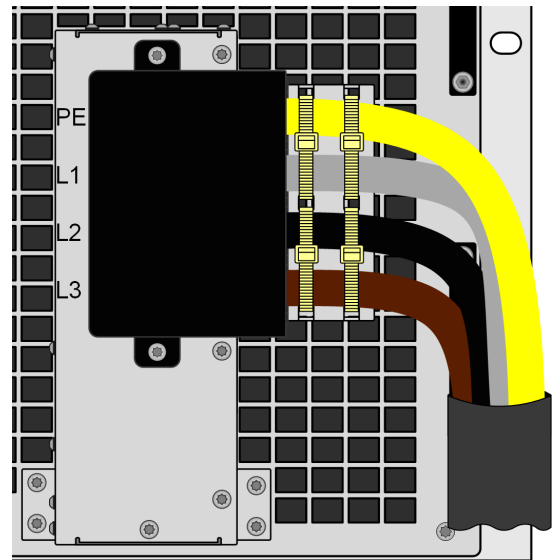
Bild 11 - Kompletter AC-Anschluß
