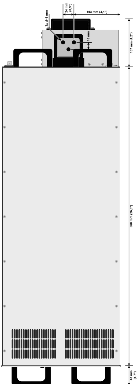
Seitenansicht der luftgekühlten Version
