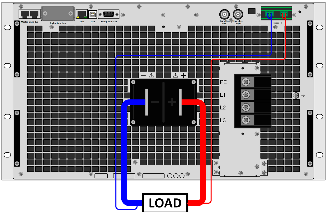
Bild 13 - Beispiel Fernfühlungsverdrahtung (DC- und Sense-Abdeckungen zu Zwecken der Veranschaulichung weggelassen)
