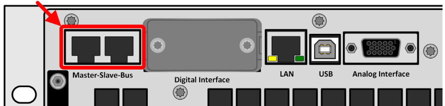
Bild 7 - Master-Slave-Busanschlüsse
