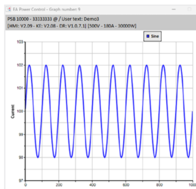
AC-Amplitude einstellbar
